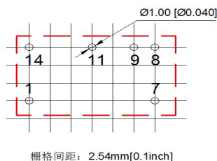
推荐 PCB 图
