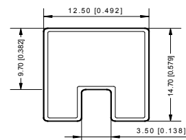
包装管尺寸图
