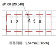
推荐 PCB 图
