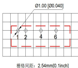
推荐 PCB 图
