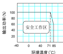
温度曲线图
