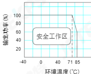
温度曲线图
