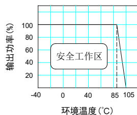
温度曲线图
