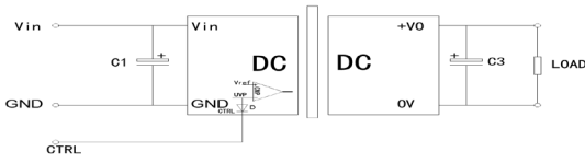
单路输出
