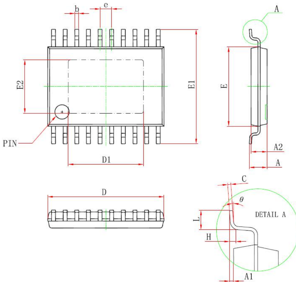
TSSOP20-PP Package
