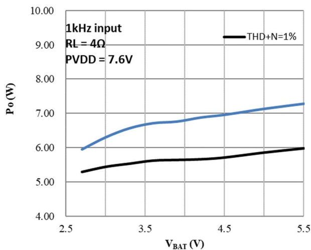
V_{BAT} vs P_o
