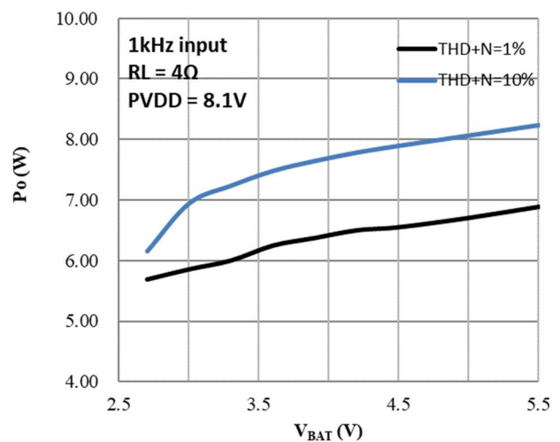
V_{BAT} vs P_o
