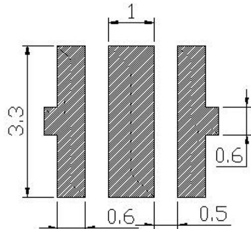
焊盘建议图
