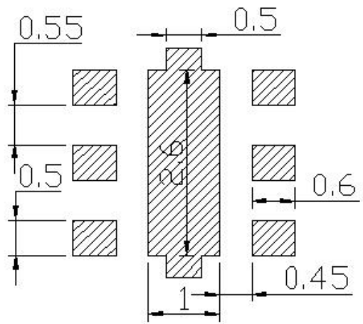
焊盘建议图
