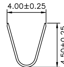
SEC:A-A
