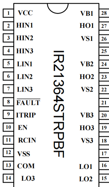
图4-1 28-脚 SOP 顶视图
