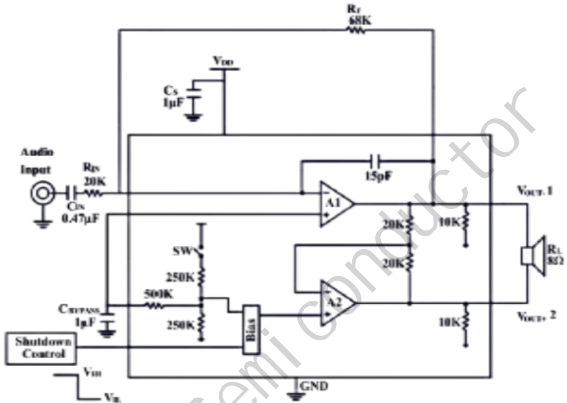
(图 1) LM4890 典型应用原理图
