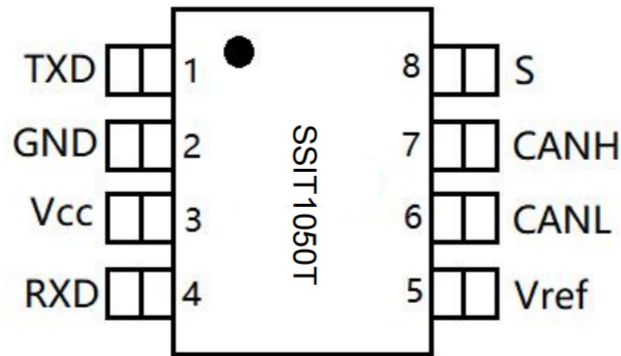
图 2: SSIT1050T引脚图
