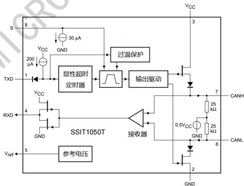
图1: SSIT1050T逻辑图
