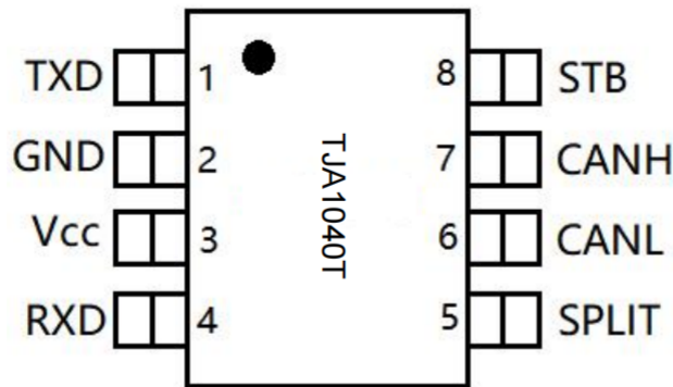
图 2: TJA1040T引脚图
