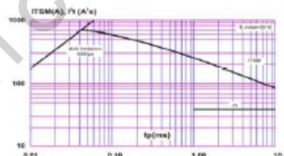
6、 I_{TSM}-t, I^2t-1 曲线
