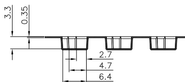
SECTION A-A SCALE 1:1
