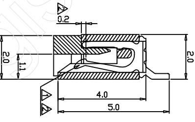
SECTION A-A 下接触
