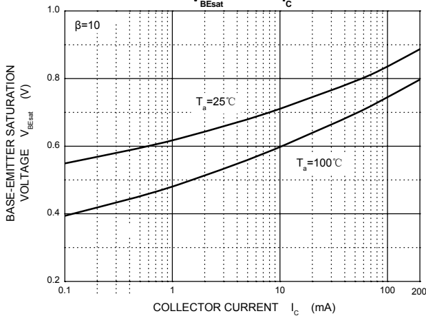
V_{BE} - I_c
