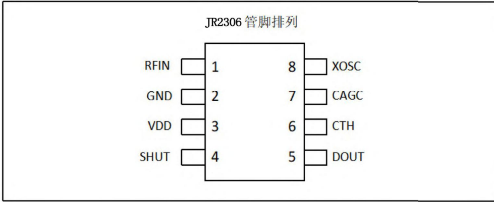
图 2 JR2306 管脚排列图
