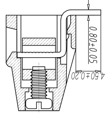
剖面图 A-A
