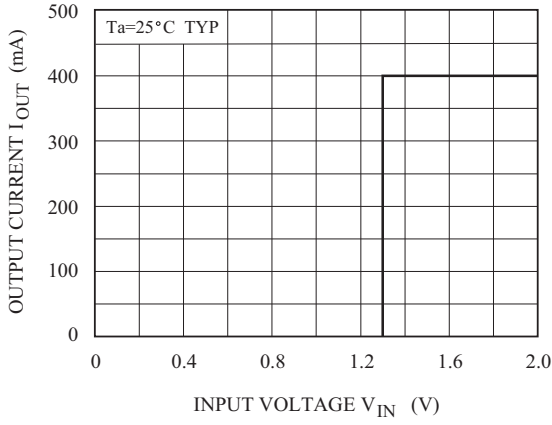
I_{OUT} - V_{IN}
