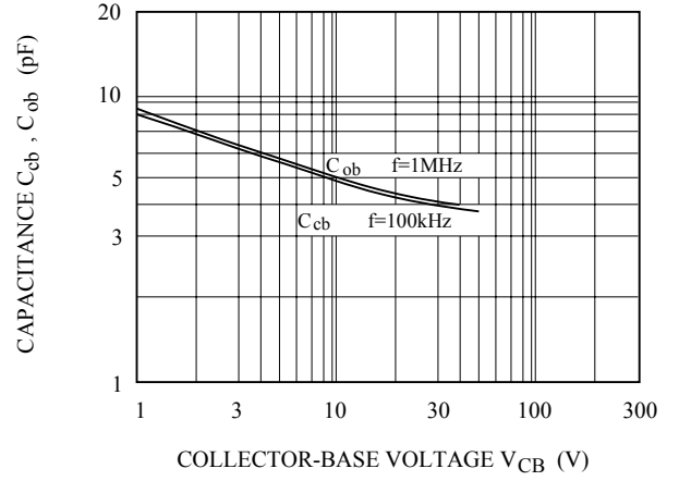
C_{cb}, C_{ob} - V_{CB}
