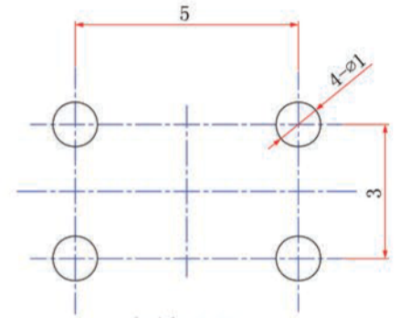
线路板孔位
