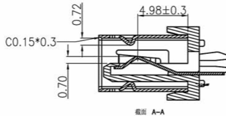
截面 A-A
