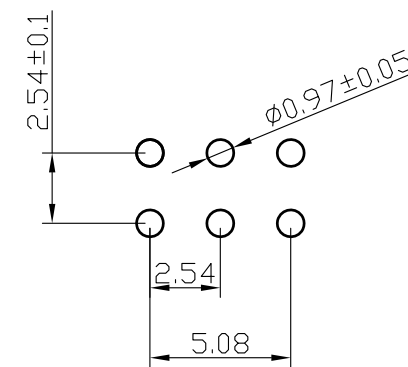
PCB开孔
