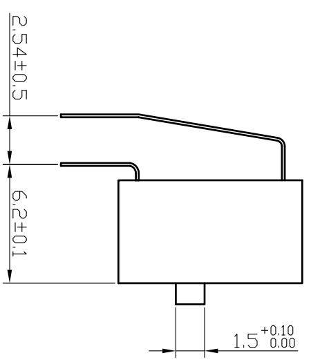
高推钮 (E)
