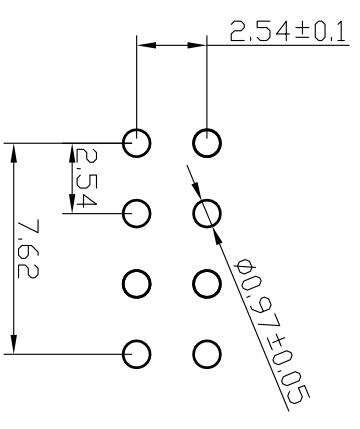
PCB开孔
