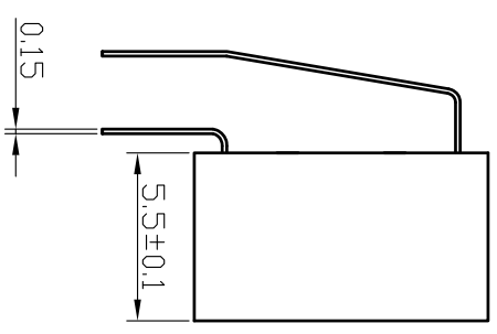
平推钮 (R)
