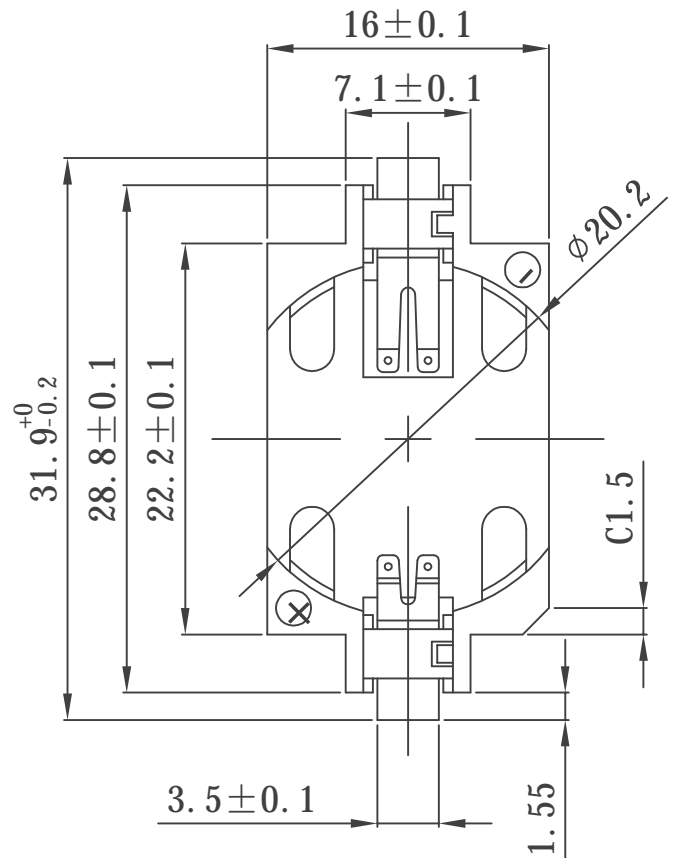
安装尺寸
