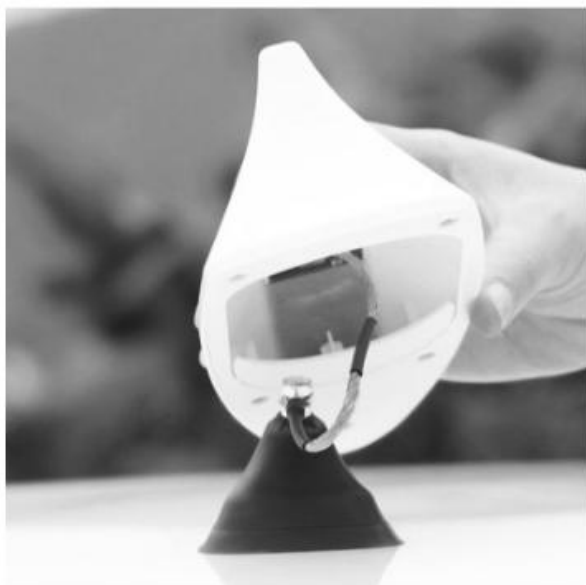
第三步：天线连接成功
