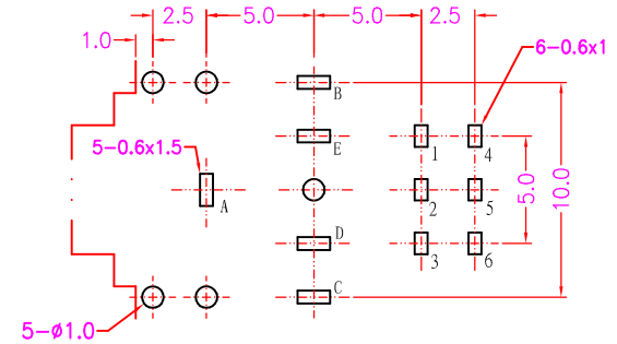
印制板开孔示意图
