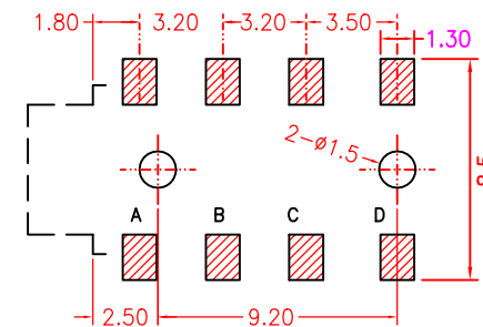
印制板开孔示意图
