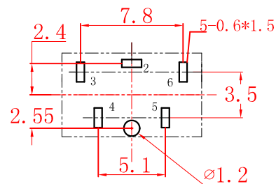
线路板开孔尺寸
