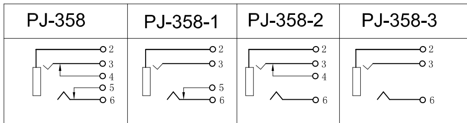
电路原理图
