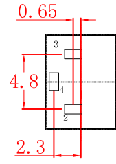
线路板开孔尺寸
