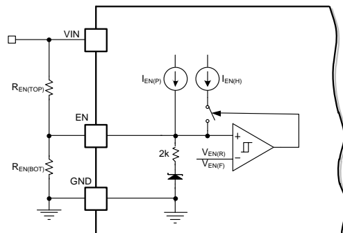
图 9-2 V_{IN} UVLO 阈值设置
