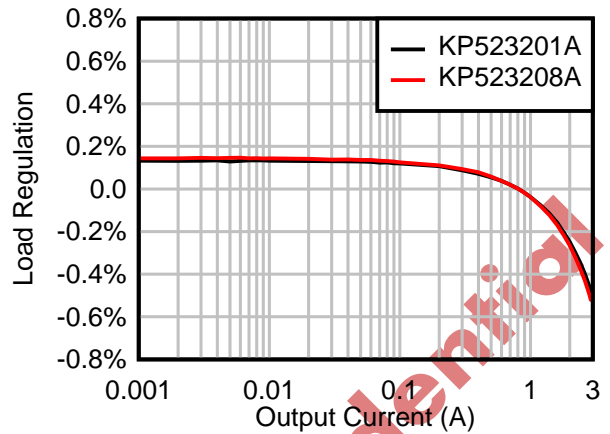
图 10-19 负载调整率 V_{OUT} = 3.3V
