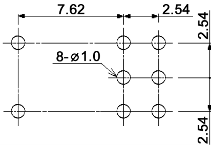
P.C. LAYOUT
