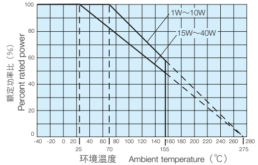
■ 负荷减轻特性曲线 Derating Curve
