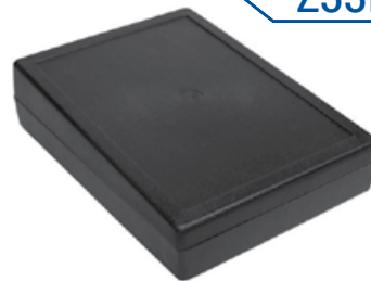
Z33B
