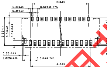
推奨パターン寸法 (2929番目) RECOMMENDED PATTERN LAYOUT
