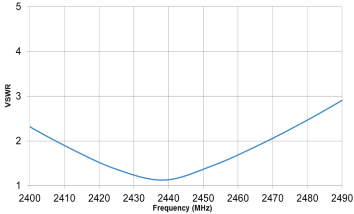
2.4 GHz VSWR
