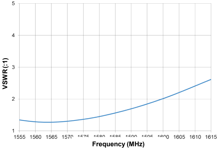
VSWR
