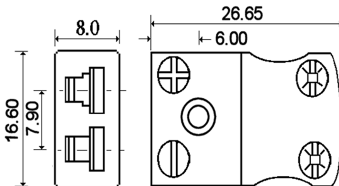
Miniature Socket
