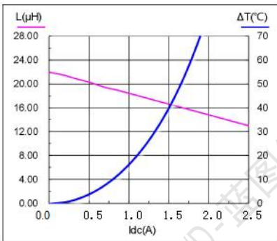
SMS0420-220M
