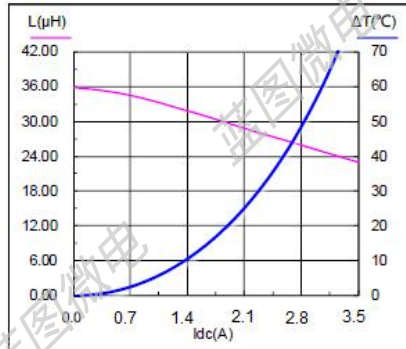
SMS0630-330M
