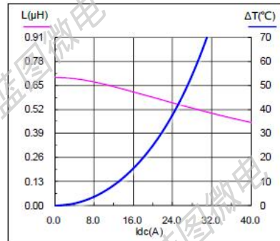
SMS1040-2R2M
