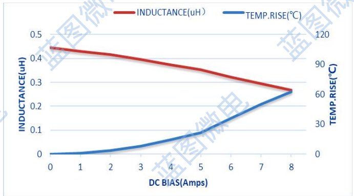
STC201610-R47M
