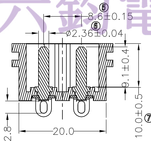
scetion A-A
