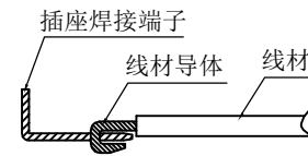
焊接(钩焊)示意图
