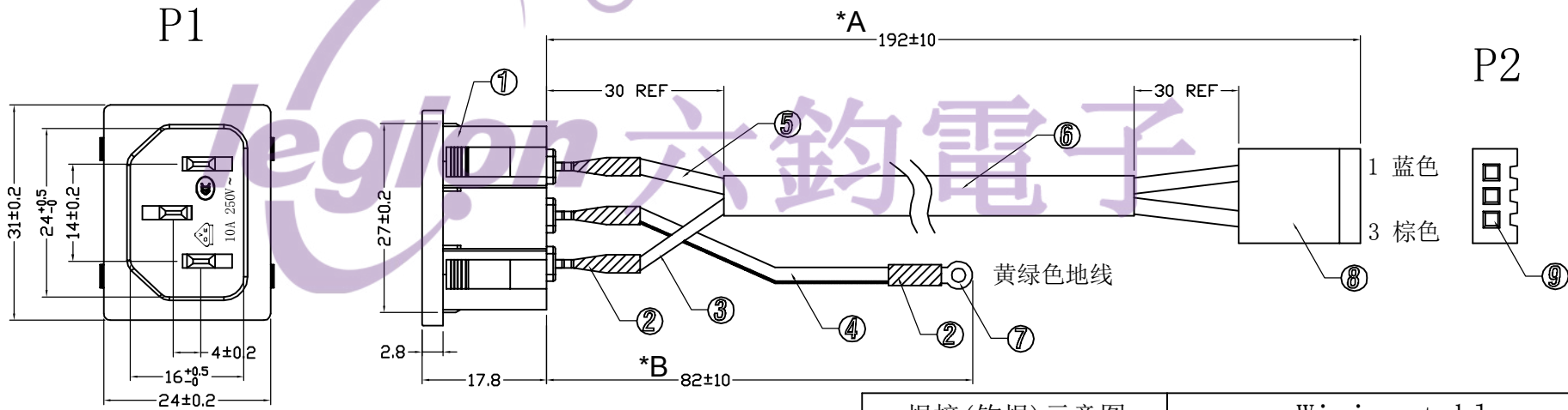
焊接(钩焊)示意图
